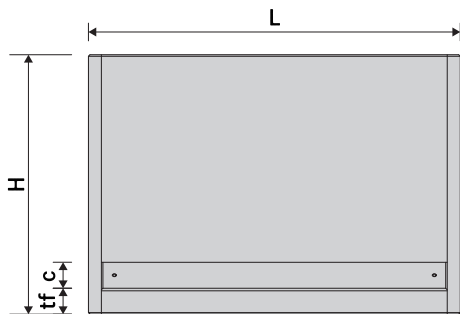
背面図
