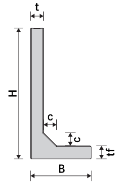
側面図
