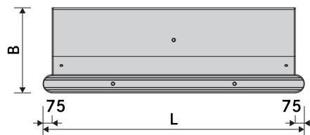
平面図
